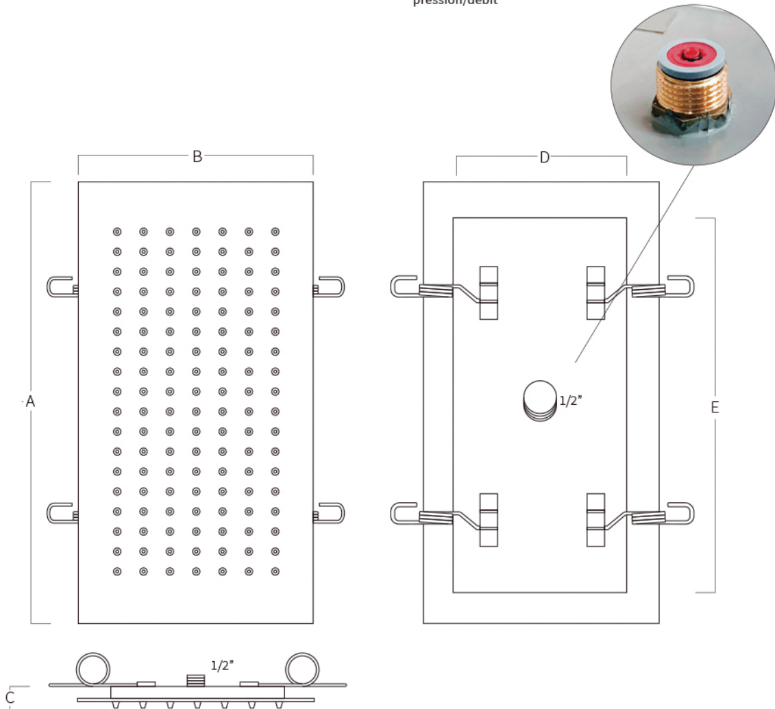
Réducteur de pression/débit
